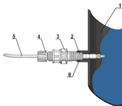
Fig. 7 - Montaggio Raccordo
