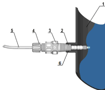
Fig. 7 - Montaje del racor
