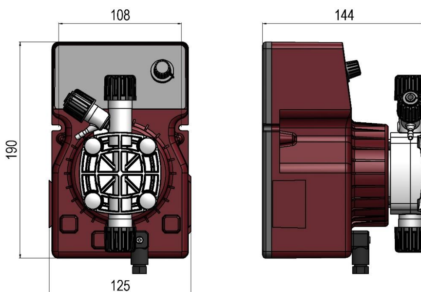
Fig. 1b – Bomba PMF, con fijación a pared (dimensiones indicadas en mm).
