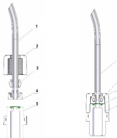
Fig.4 – Conexión hidráulica
