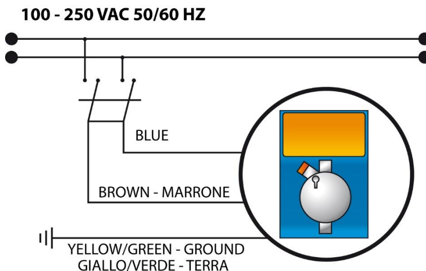
Abb. 3 – Anschluss an die Stromversorgung
