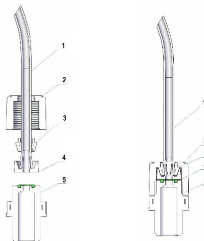
Fig.4 – Collegamento idraulico
