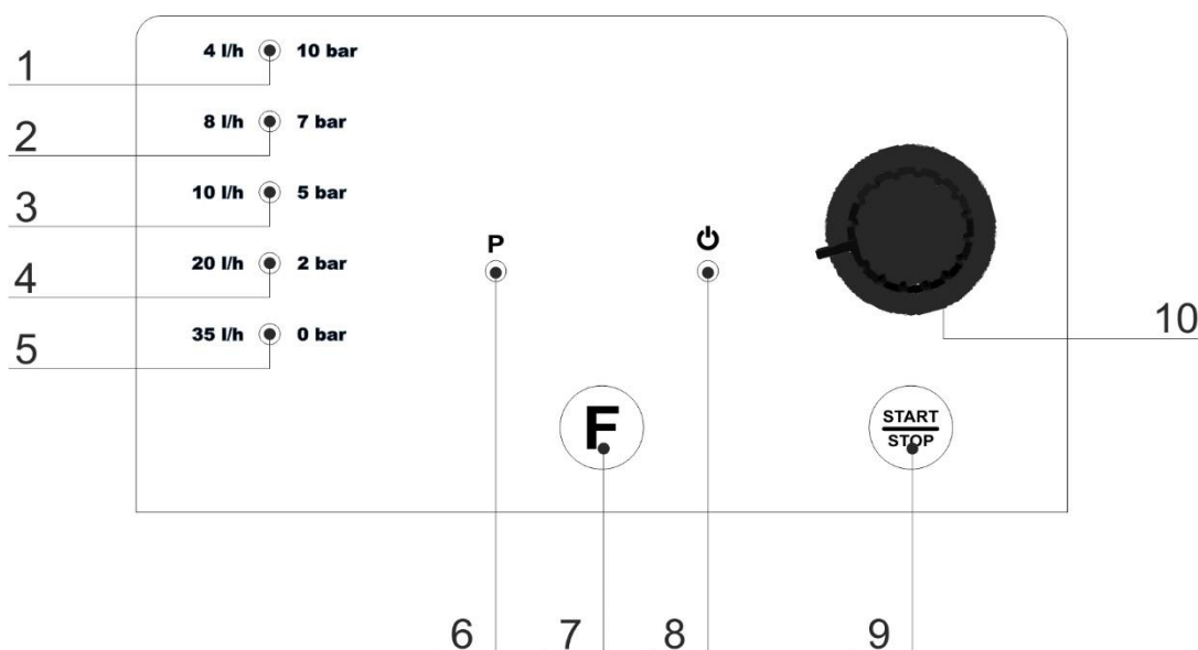
Fig. 8 - Panel de mandos y señalización
