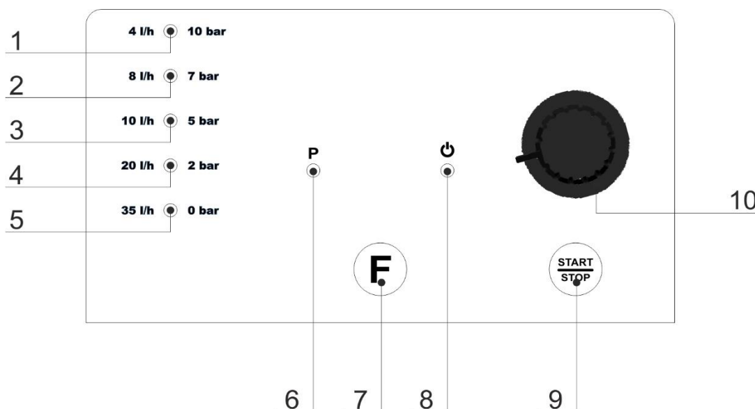
Fig. Fig.8 - Panneau de commande et de signalisation
