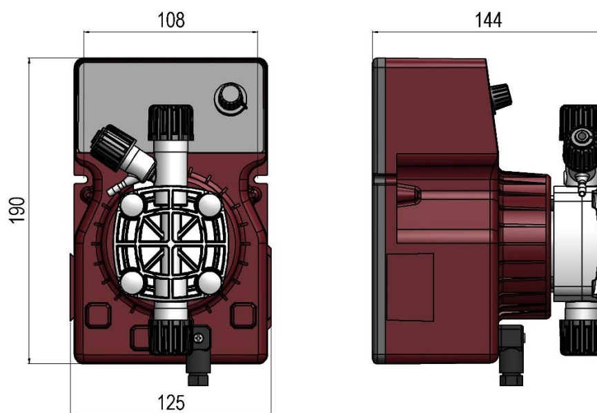
Abb. 1b – Pumpe PMF, Wandmontage (Abmessungen in mm).
