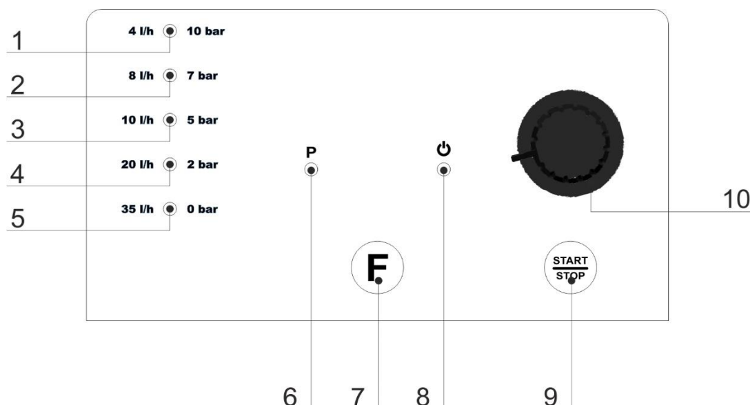
Fig. 8 - Pannello comandi e segnalazione
